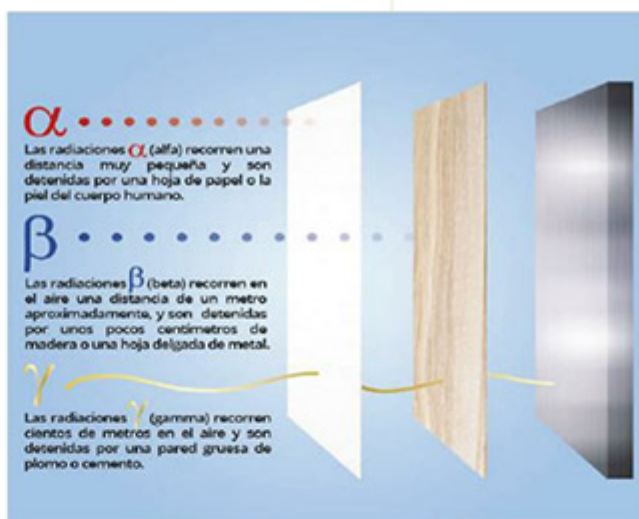
FIGURA 2. TIPOS DE PARTÍCULAS Y GRADO DE PENETRACIÓN. TOMADO DE: HTTP://WWW.MADRIMASD. ORG/BLOGS/CIENCIANU- CLEAR/2006/12/01/53391.
